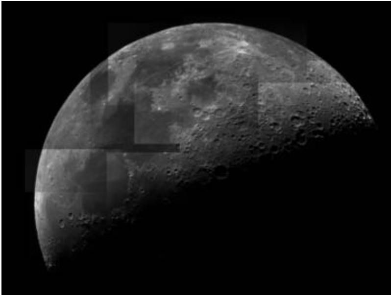
Der Mond
