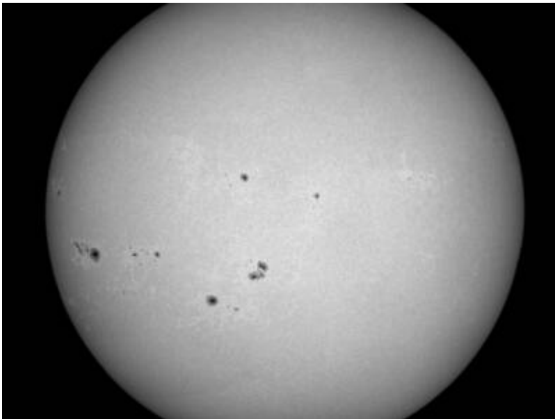
Sun
