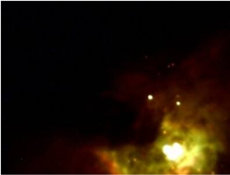
M 42 - Orionnebel
