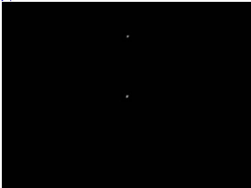
Jupiter
