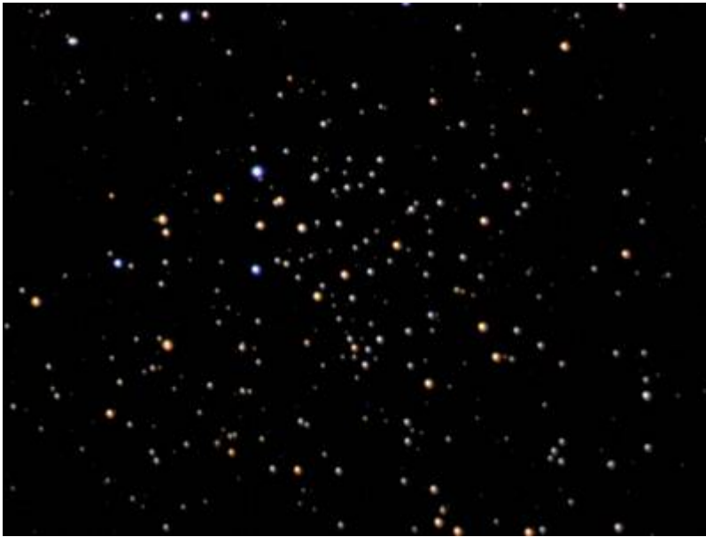
NGC 6939
