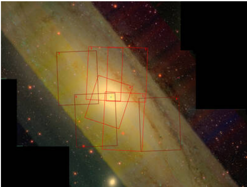
M31 - Mosaik
