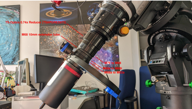
APO mit Reducer, QHY600 mit Filterrad und Off-Axis-Guider, und allen nötigen Adaptern
