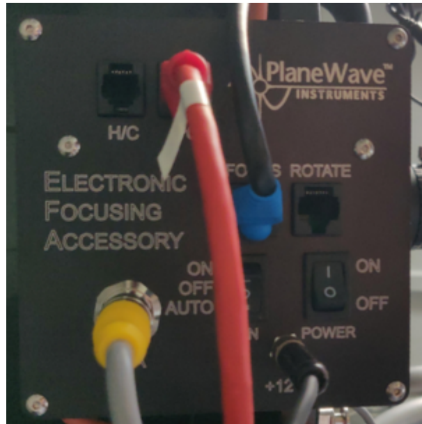
Abb. 2: Die Kontrollbox des Okularauszugs
